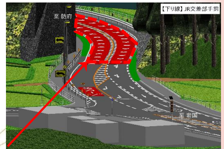
舗装改修箇所（切削オーバーレイ・カラー舗装・区画線）
