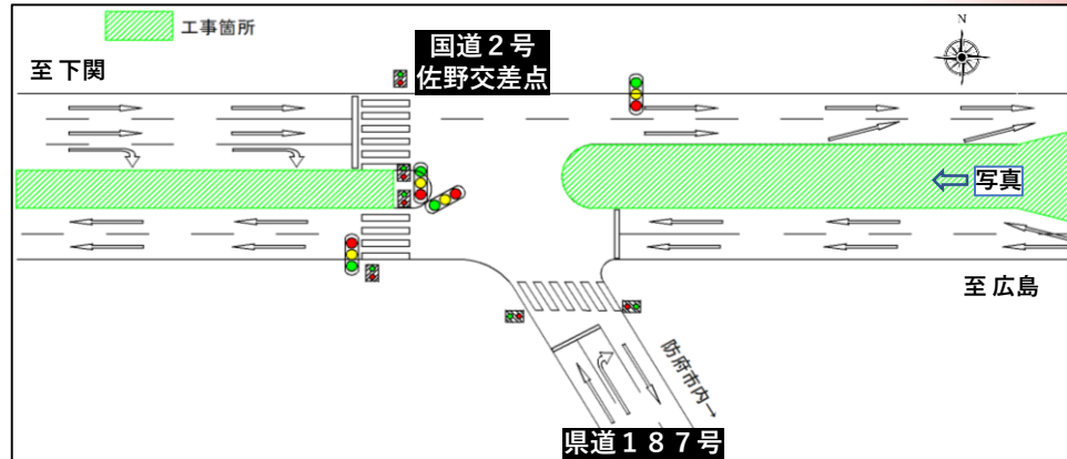
佐野交差点下り線切替図
