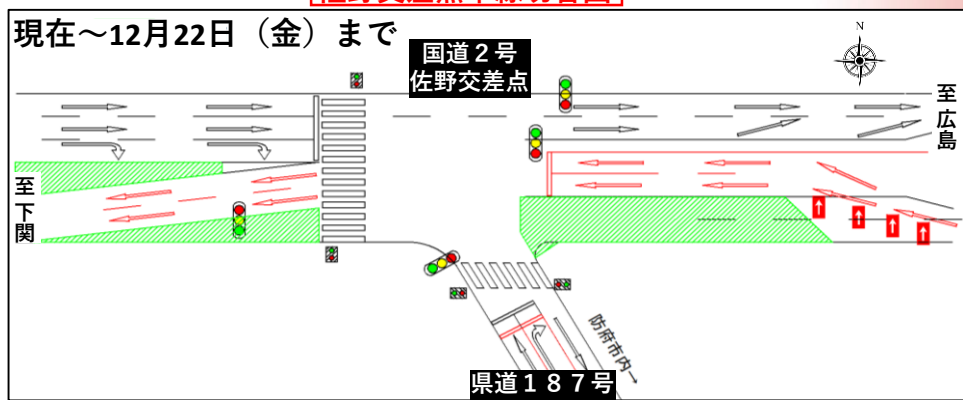
佐野交差点車線切替図
