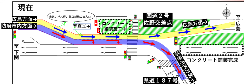
佐野交差点車線切替図
