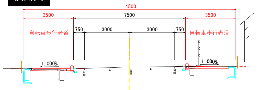
横断面
