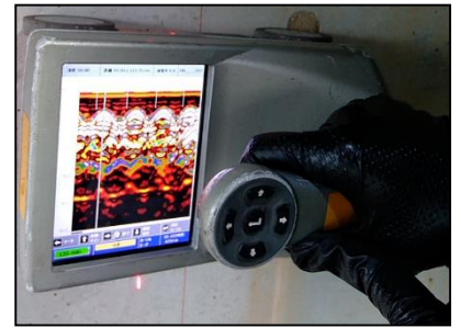
▲探査状況 (鉄筋探知デモンストレーション)
