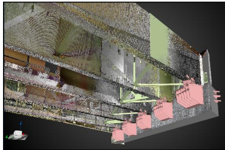
▲既設橋と耐震補強構造のモデル化
