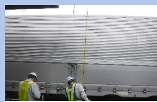
車両寸法計測（高さ）
