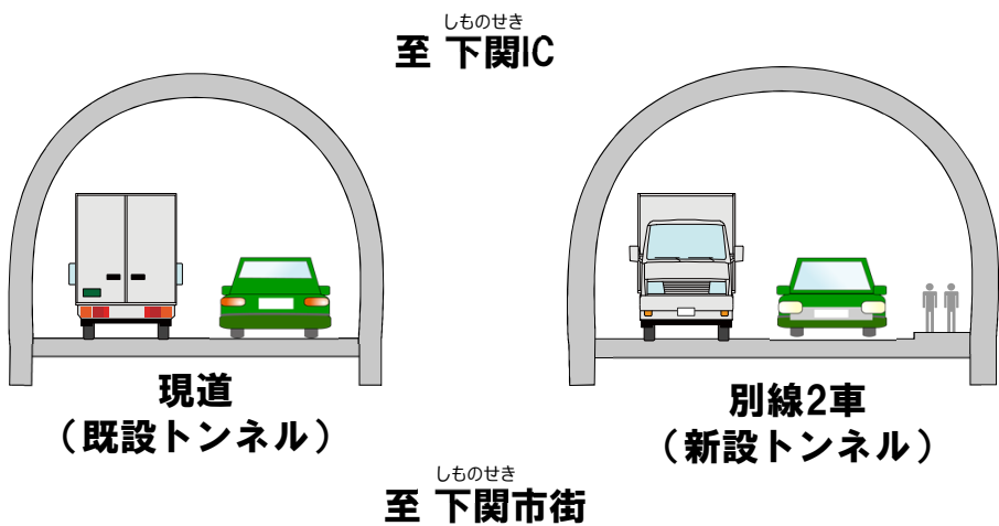
横断面図
