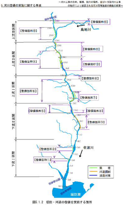
図5.1.2 堤防・河道の整備を実施する箇所
