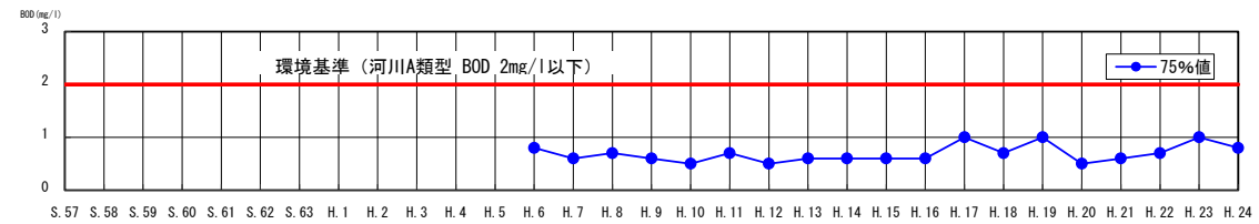
BODの経年変化（堀）
