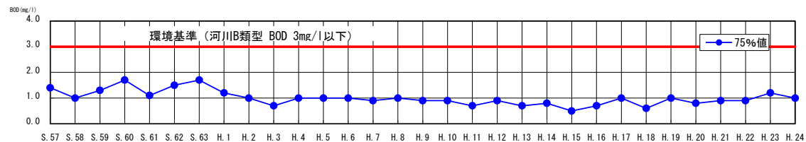
BODの経年変化（佐波川大橋）
