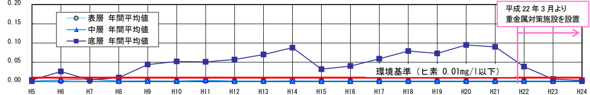
重金属類（ヒ素）の経年変化（島地川ダム堰堤直上流）
