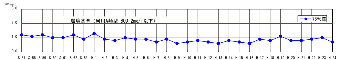
BODの経年変化（新橋）
