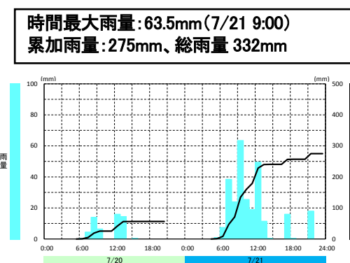
図 2.2.3 防府観測所雨量（気象庁）
