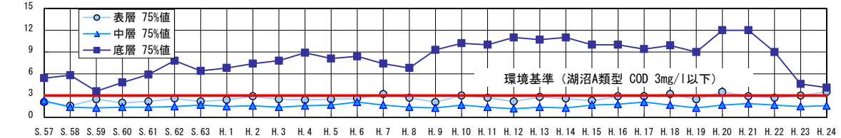
CODの経年変化（島地川ダム堰堤直上流）
