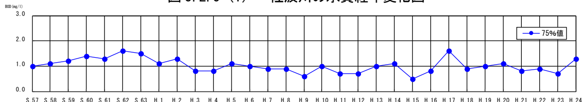
BODの経年変化（和田）
