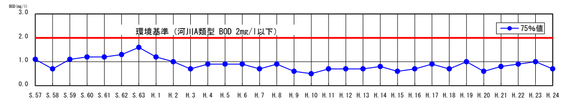
BODの経年変化（漆尾）
