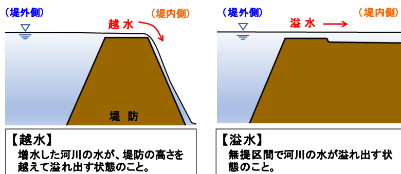
図9 越水と溢水
