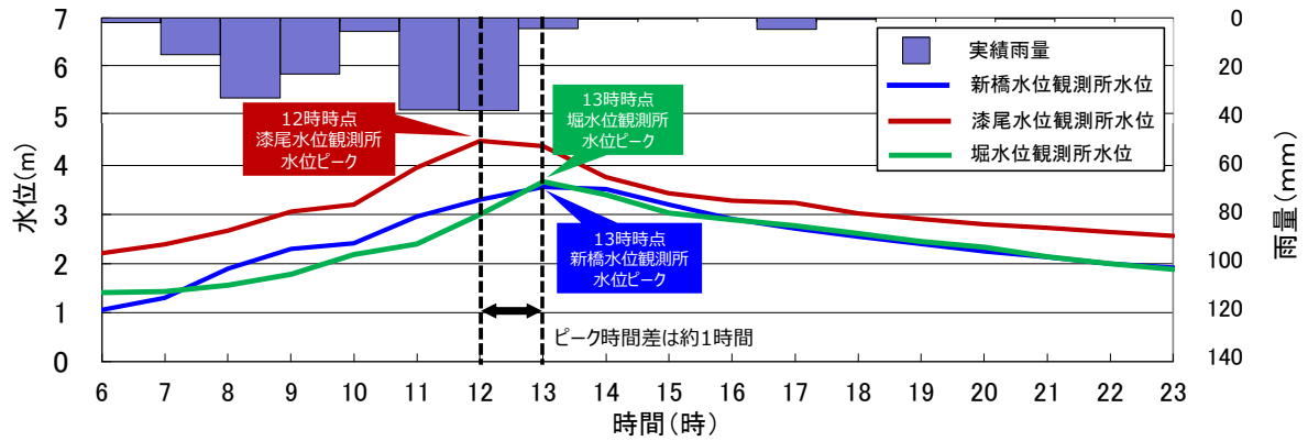
図 5-3 平成 21 年 7 月洪水における各水位観測所の水位上昇（平成 21 年 7 月 21 日観測）
