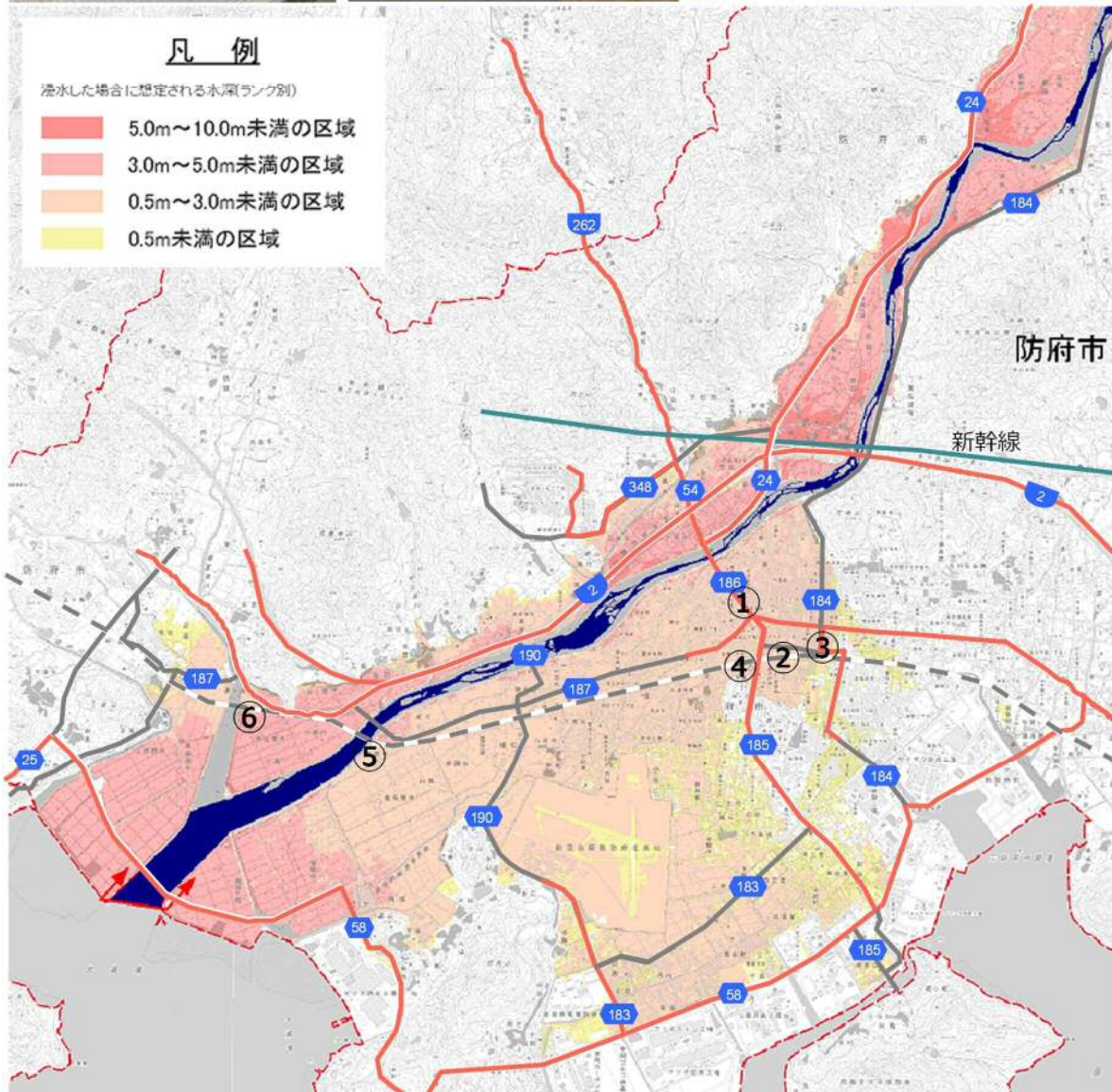
図 2-2 佐波川洪水浸水想定区域図 (想定最大規模)
