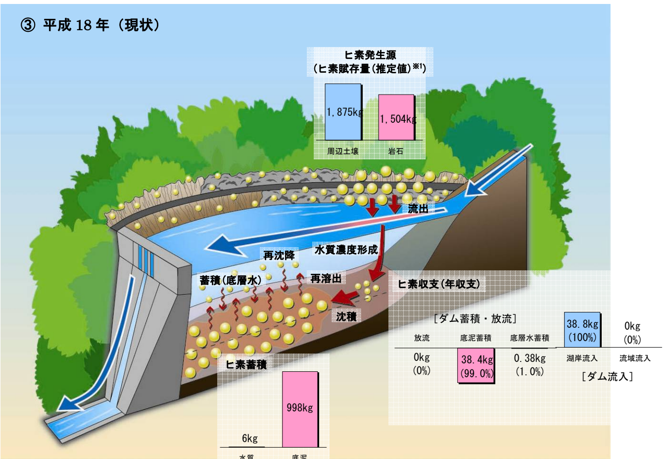
図 3.3-3(2) 島地川ダム湖のヒ素汚染メカニズム模式図
