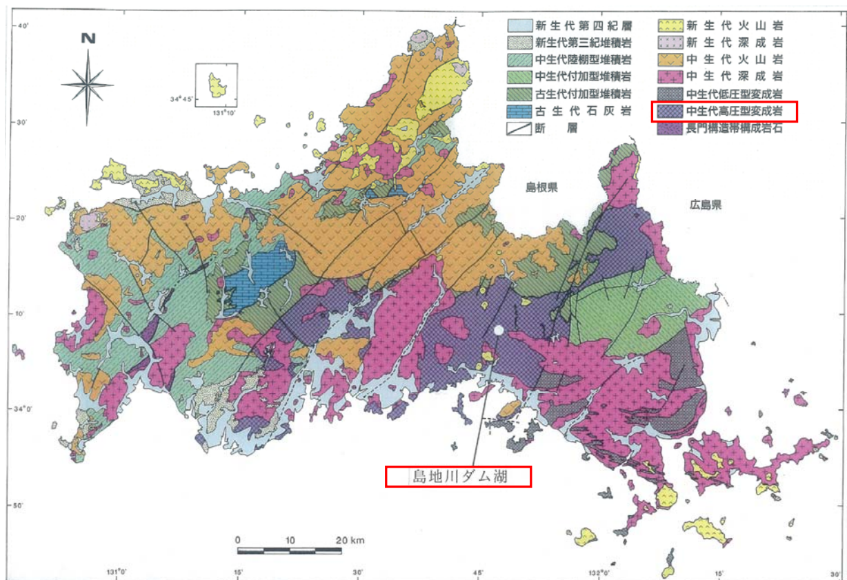
図 1-5 (1) 山口県の地質図 (山口県地学会・編者代表 西村祐次郎・松里英男：山口県の岩石図鑑)
