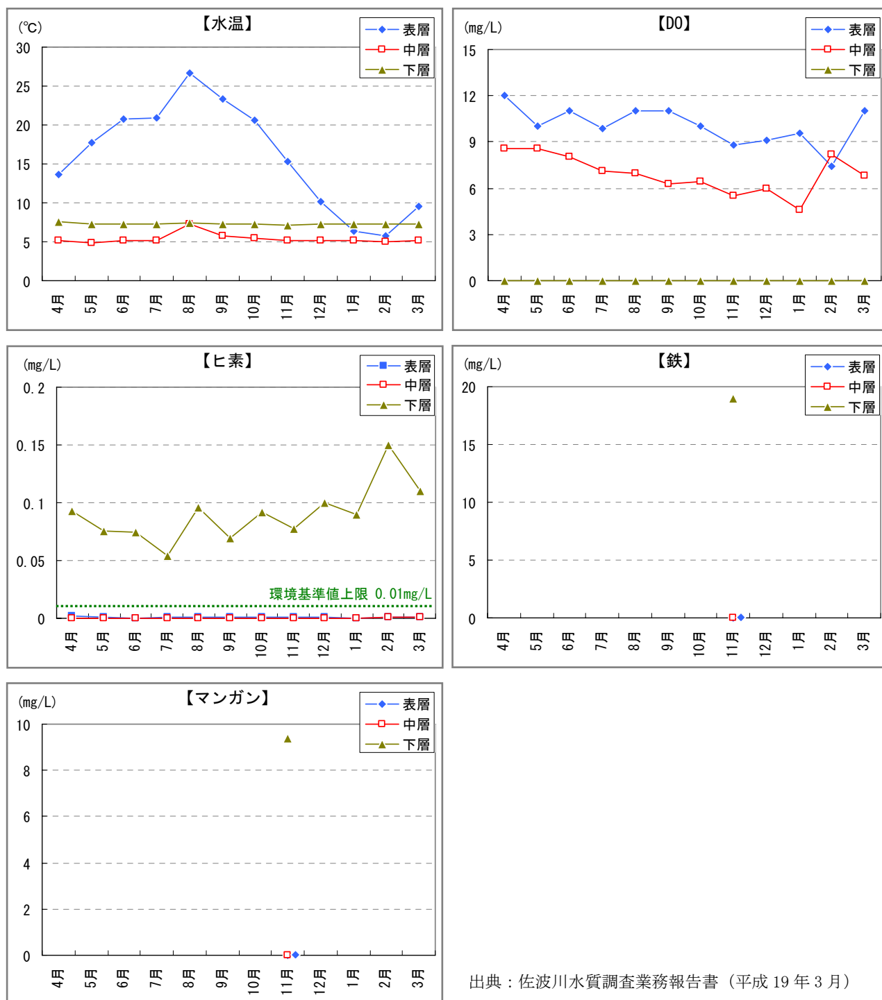
図 1-7 底層水質の季節変化（平成 18 年度，M1） （項目：水温，DO，ヒ素，Fe，Mn）
