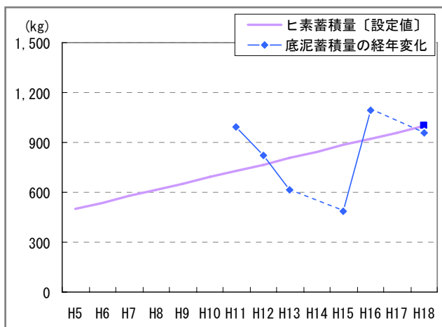
図 3.2-4 底泥のヒ素蓄積量の経年変化
