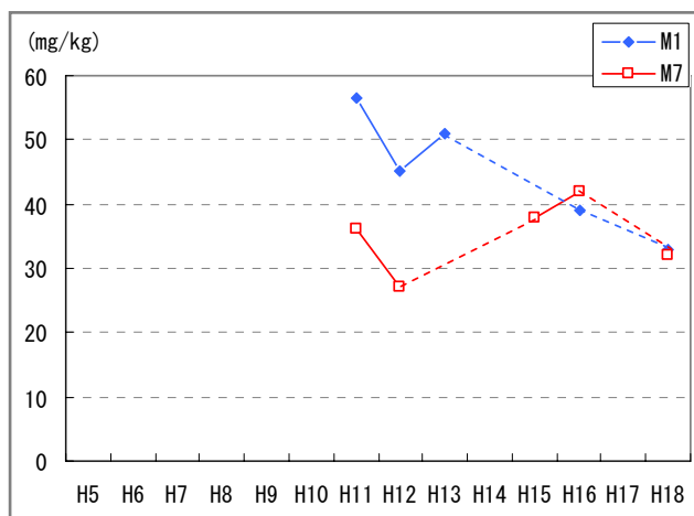
図 3.2-3 底質のヒ素含有量経年変化（M1，M7）
