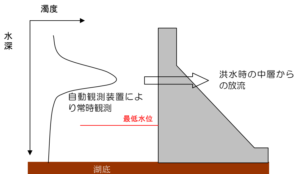
図 1-6 選択取水設備側面図
