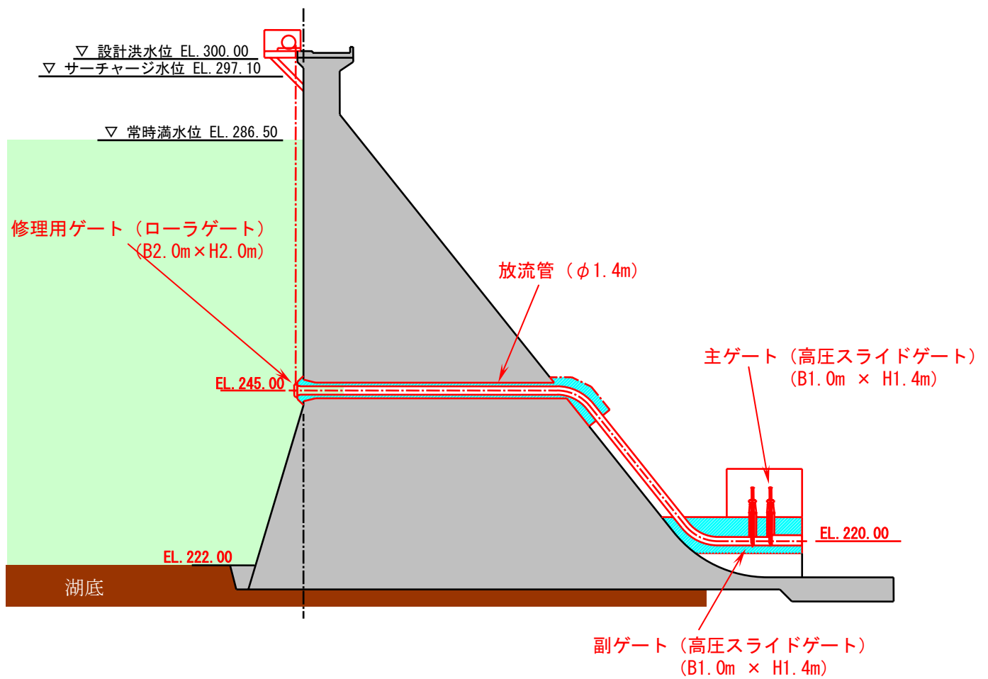
図 1-4 環境放流管
