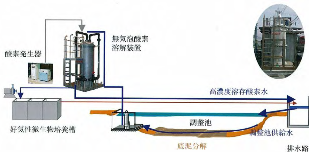
図 1-12 システム概要（メーカーパンフレットより）
