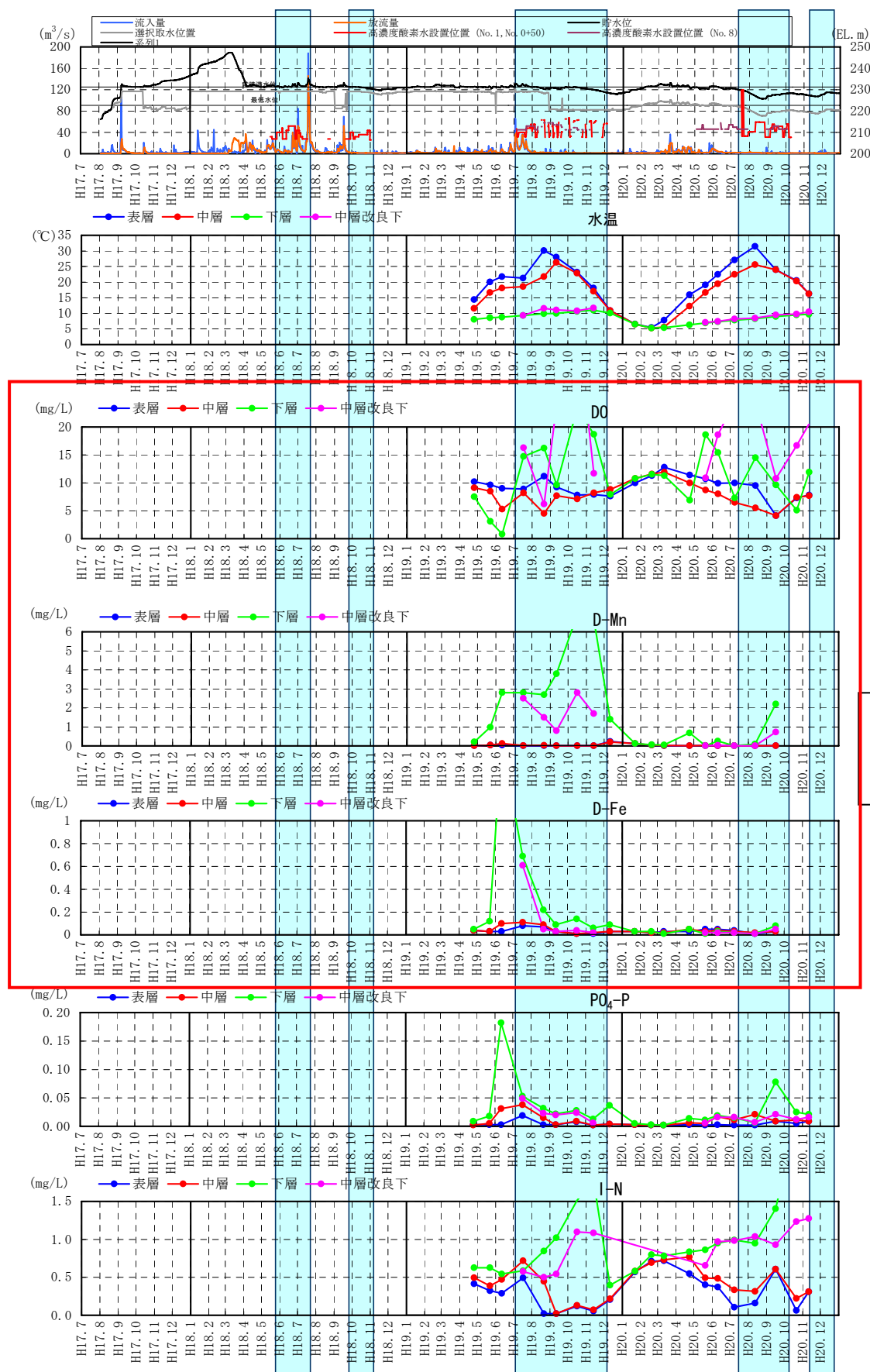
図 3-8 灰塚ダム : No. 7 の経日変化
