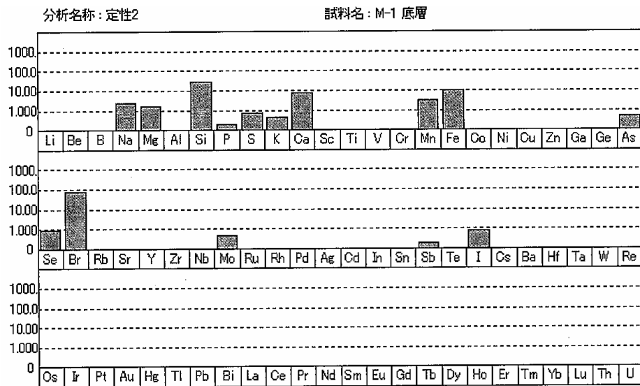
図 1-3 ICP 発光分光分析法による分析結果
