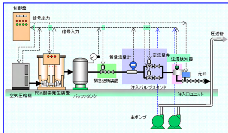
図 1-15 システム概要（メーカーウェブサイトより）
