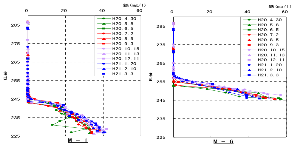
図 1-7 鉄の鉛直分布 (平成 20 年度)
