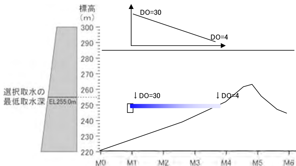
図 3-6 酸素濃度の仮定
