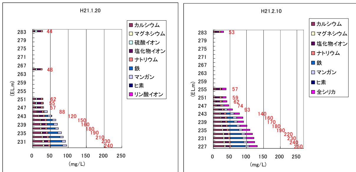
図1-1 蒸発残留物及び金属類等の鉛直分布
