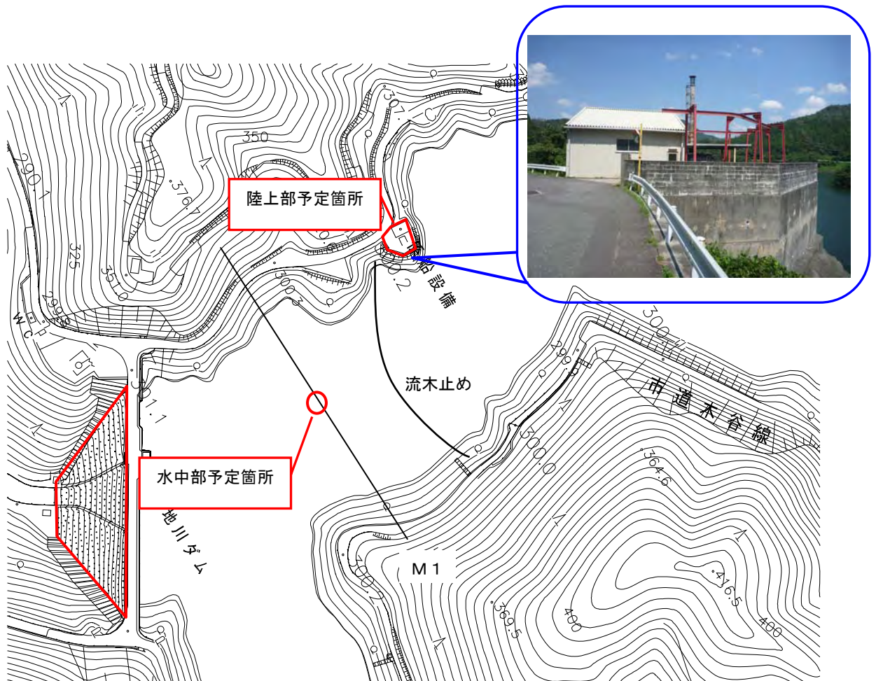
図 2-2 水中部及び陸上部の設置箇所
