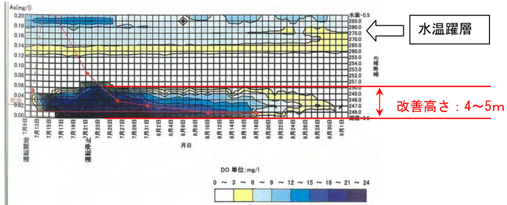
図 3-5 M-6におけるDOの改善効果（装置下流 50m）
