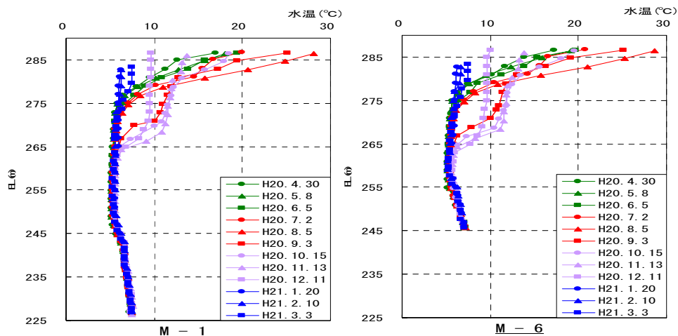
図 1-4 水温の鉛直分布（平成 20 年度）
