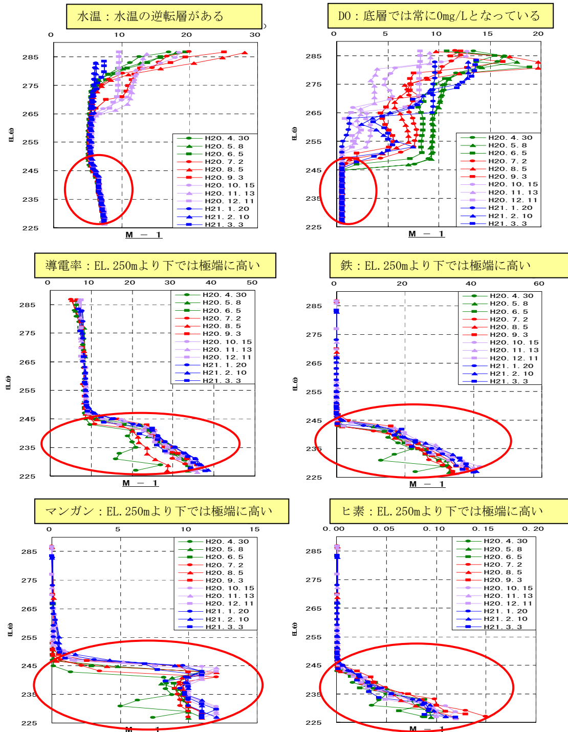
図 3-2 水質の鉛直分布（平成 20 年度, M1）
