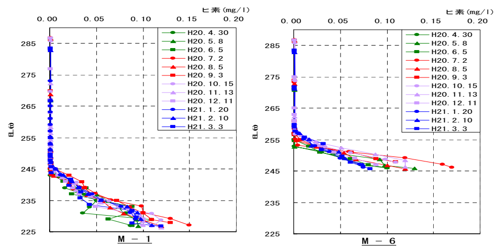
図 1-9 ヒ素の鉛直分布 (平成 20 年度)
