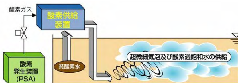
図 1-13 システム概要（メーカーパンフレットより）
