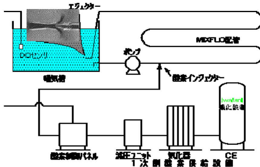
図 1-14 システム概要（メーカーウェブサイトより）
