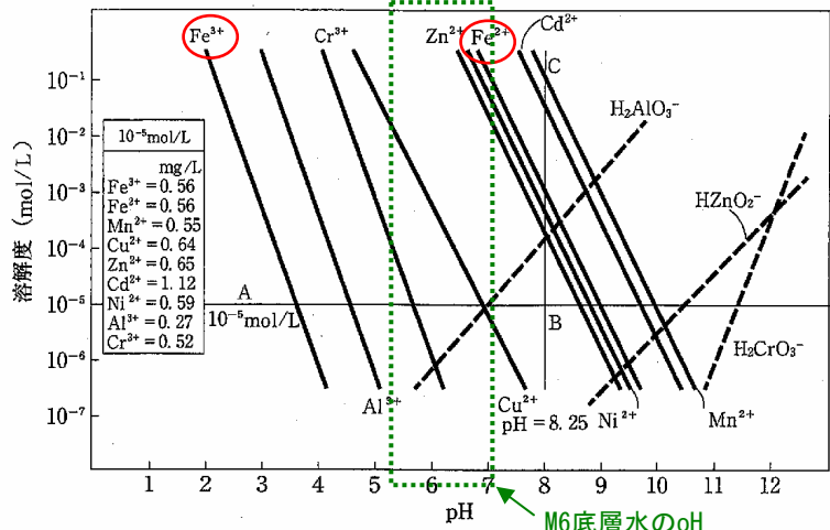
図 1-10 pHと金属類の溶解度の関係
