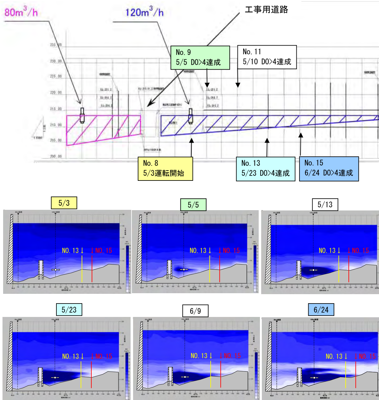
図 3-7 灰塚ダム NO. 8 における酸素の到達状況
