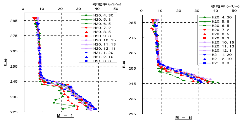
図 1-6 導電率の鉛直分布（平成 20 年度）
