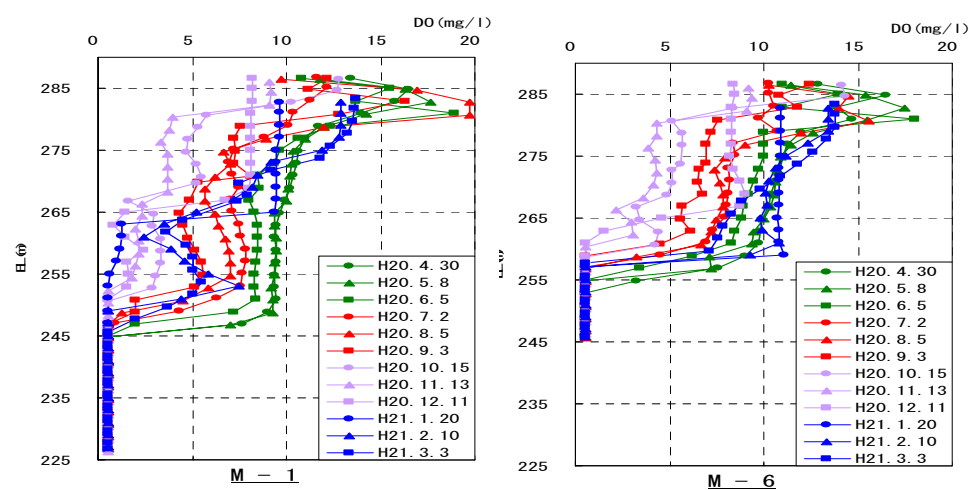
図 1-5 DO の鉛直分布（平成 20 年度）
