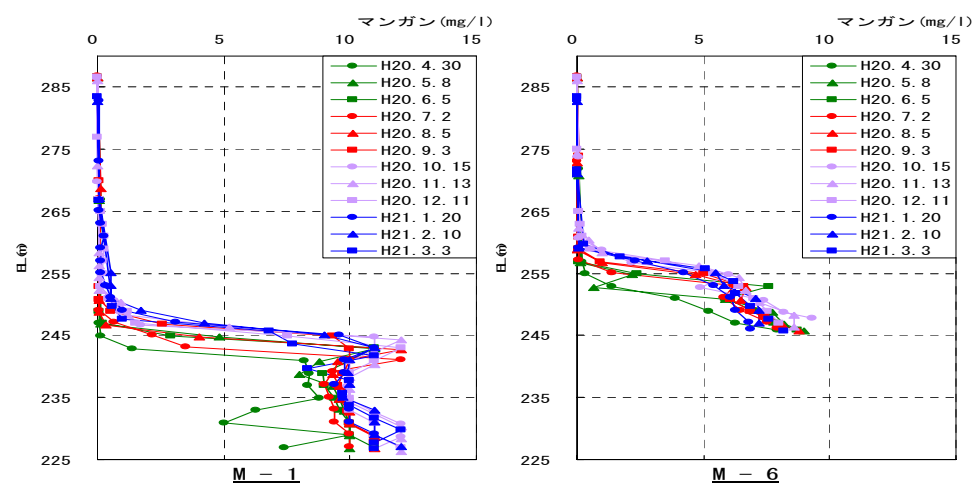
図 1-8 マンガンの鉛直分布 (平成 20 年度)
