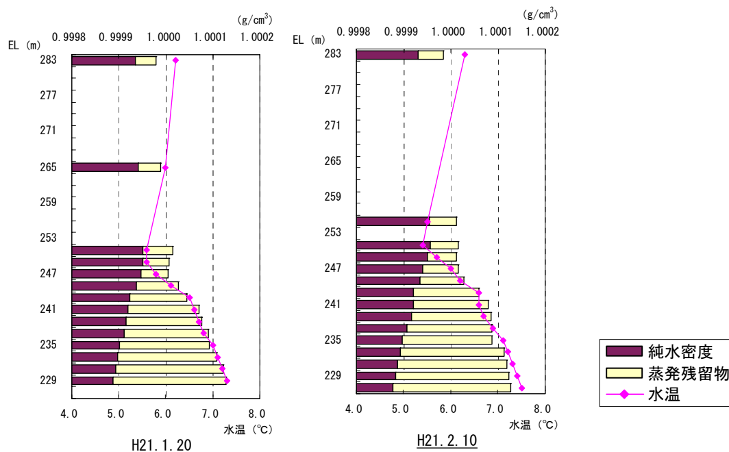
図1-2 水の密度及び蒸発残留物の鉛直分布
