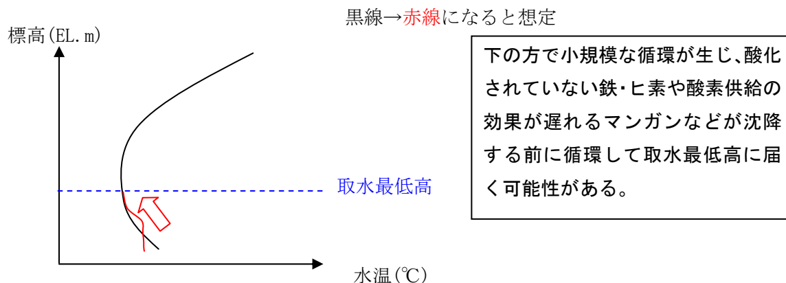
図 3-4 下から改善していく場合の水温勾配の変化イメージ
