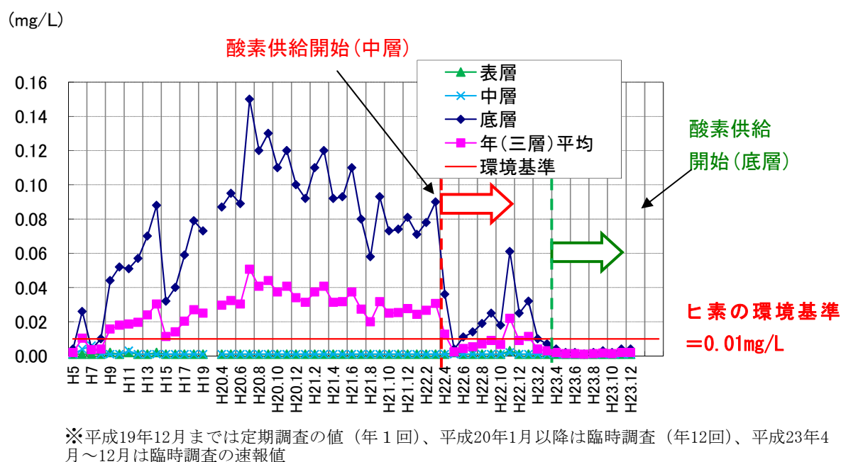
図 2-1 ヒ素の経年変化
