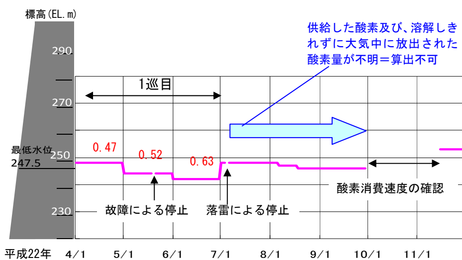
図 2-29 酸素供給開始直後の酸素消費速度
