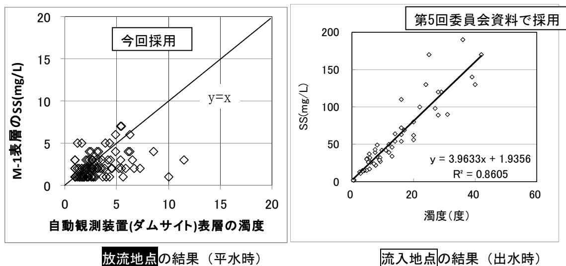
濁度とSS濃度の関係
