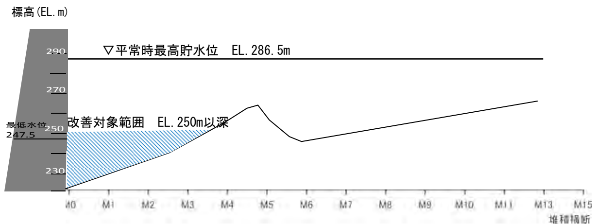
図 1-4 改善対象範囲（縦断面図）
