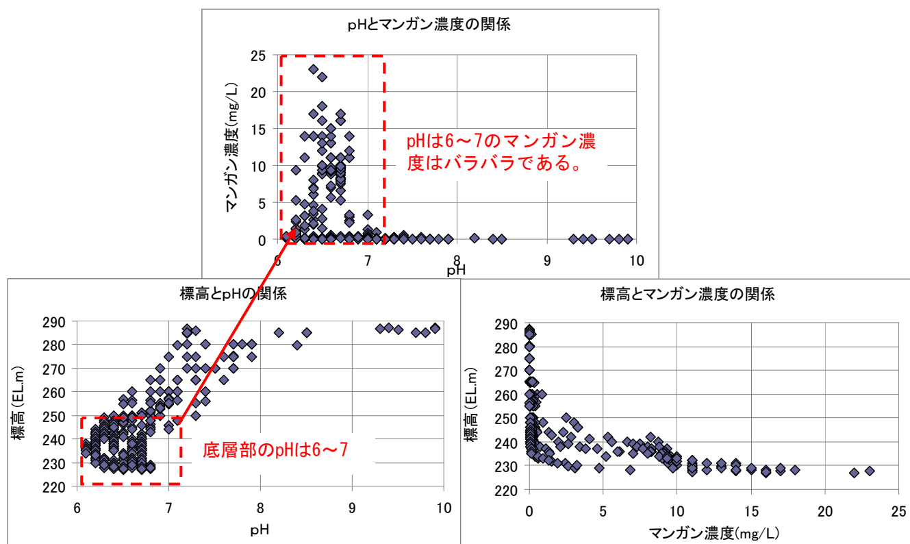
図2-35 pHとマンガン濃度及び標高の関係
