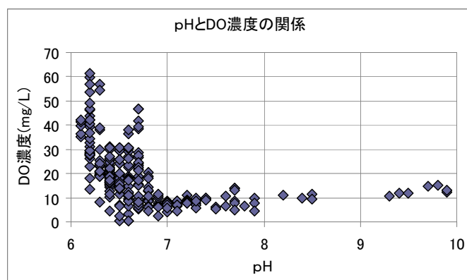
図2-36 pHとD0の関係
