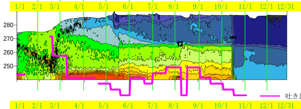
図 1-3 自動観測装置による水質の連続観測結果 (M-1 : ダムサイト)
