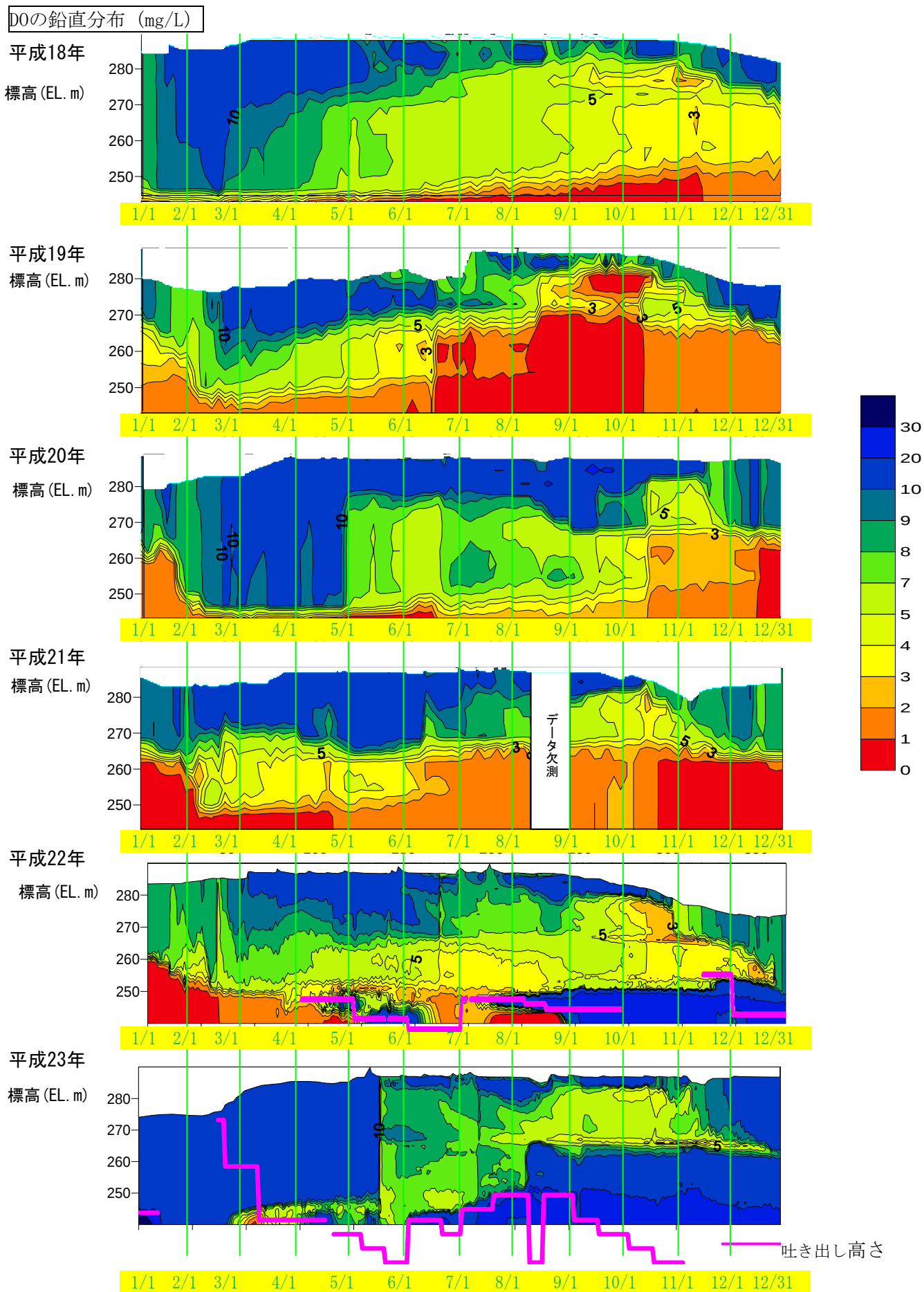
図 1-2 自動観測装置による水質の連続観測結果 (M-1 : ダムサイト)
