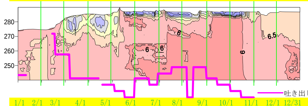
図 1-5 自動観測装置による水質の連続観測結果 (M-1 : ダムサイト)
