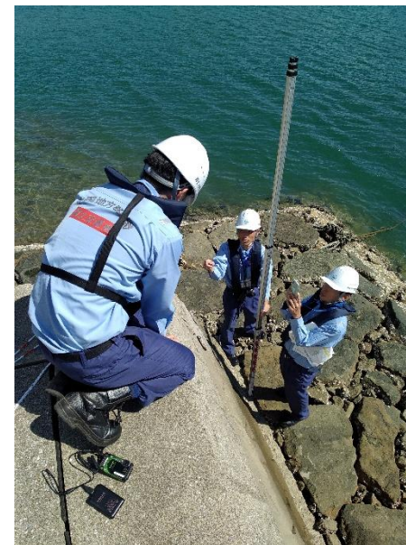
被災状況調査の状況（一町田地区）
