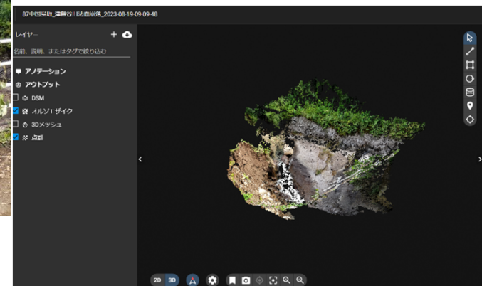
被災箇所の点群データ取得、 崩落部分の3D化
