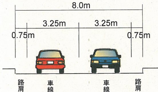
▲国道9号(現道)標準横断面図
