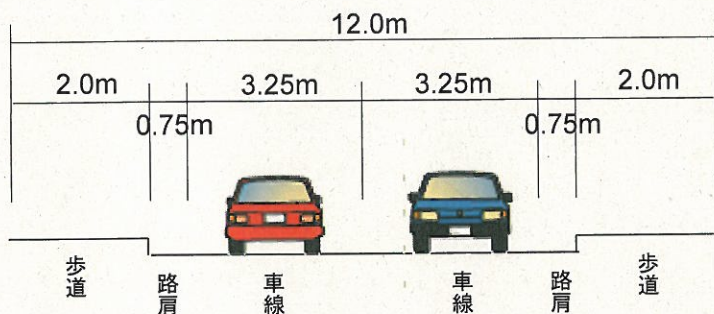
▲国道9号(現道)標準横断面図
