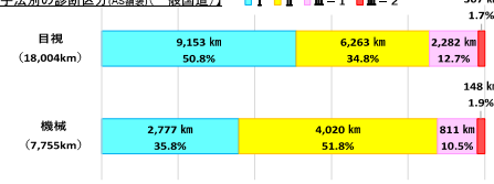
【点検手法別の診断区分(AS舗装)(一般国道)】
