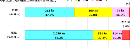
【点検手法別の診断区分(AS舗装)(自専道)】
