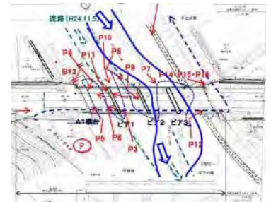
流路の変化
