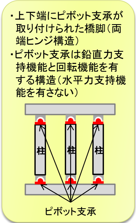
図-2 ロッキング橋脚
