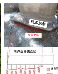
橋脚の洗掘
