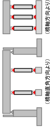
ロッキング橋脚の例
