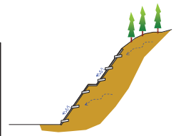
切土・斜面安定施設のイメージ
