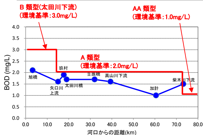
(1) BOD の変化
