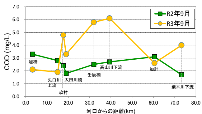
(2) COD の変化
