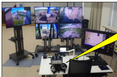
遠隔操縦装置 (モニター、リモコン)
