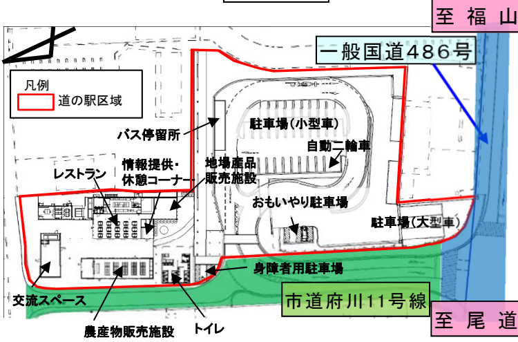
平面図
