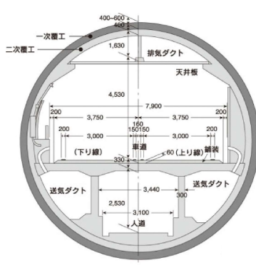
断面図(海底部)
