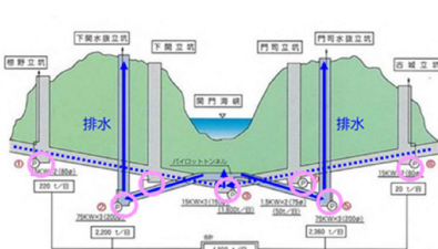
排水設備（水抜ポンプ）
