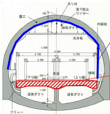
断面図（陸上部）
