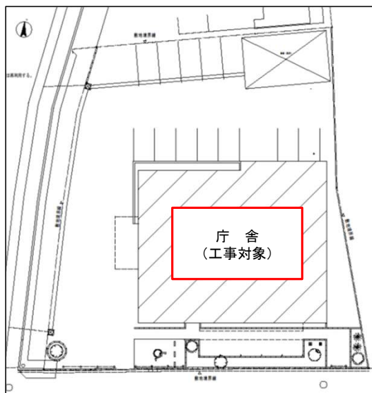
配置図
