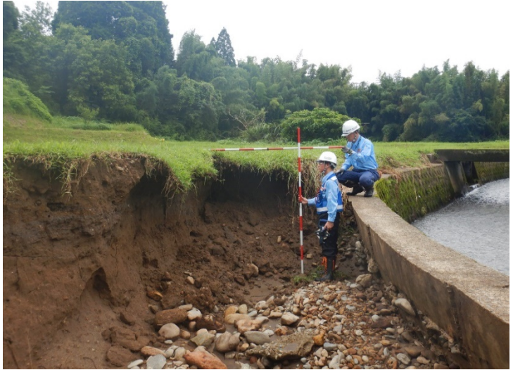
河川護岸被災箇所の現地調査（熊本県人吉市）
