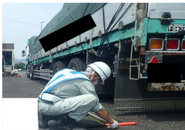
車両長計測
