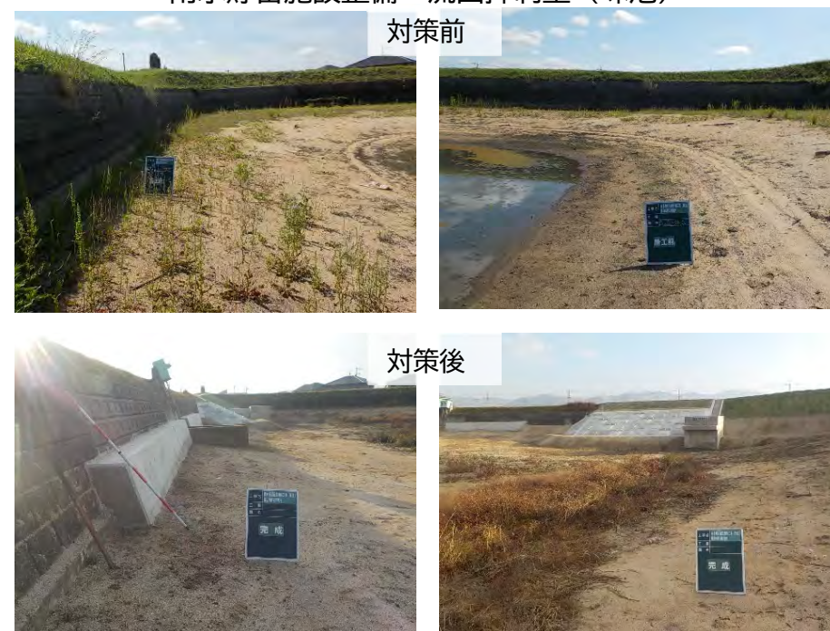
雨水貯留施設整備 流出抑制型（珠池）
