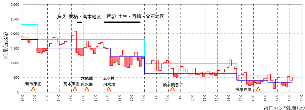
図 5-1-2 流下能力図
