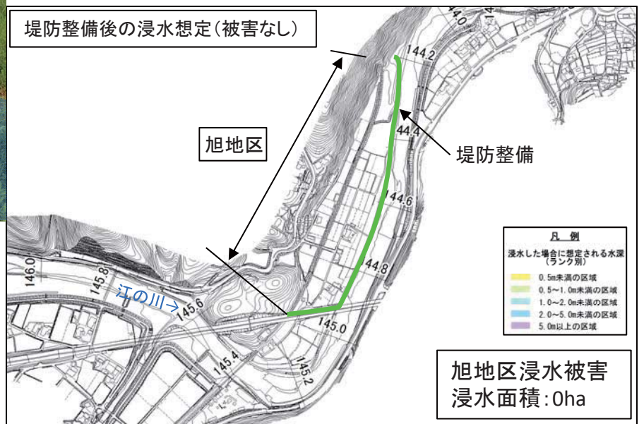
堤防整備
