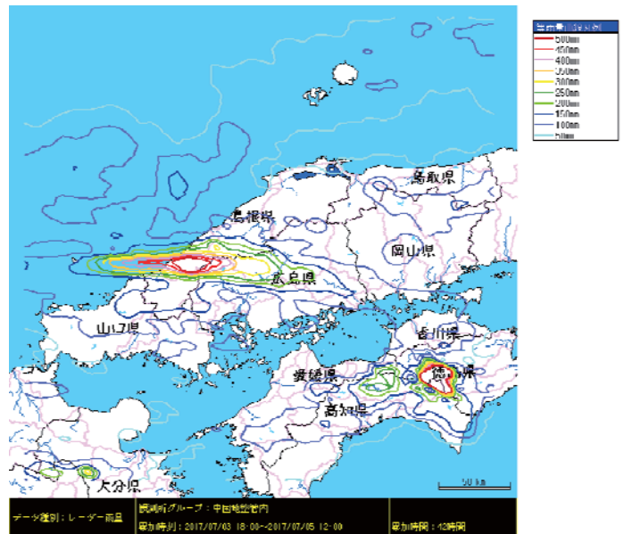
等雨量線図
