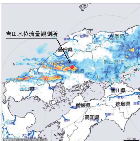
線状降水帯の状況(XRAIN)
