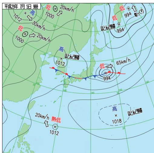
天気図(7月5日9時)
