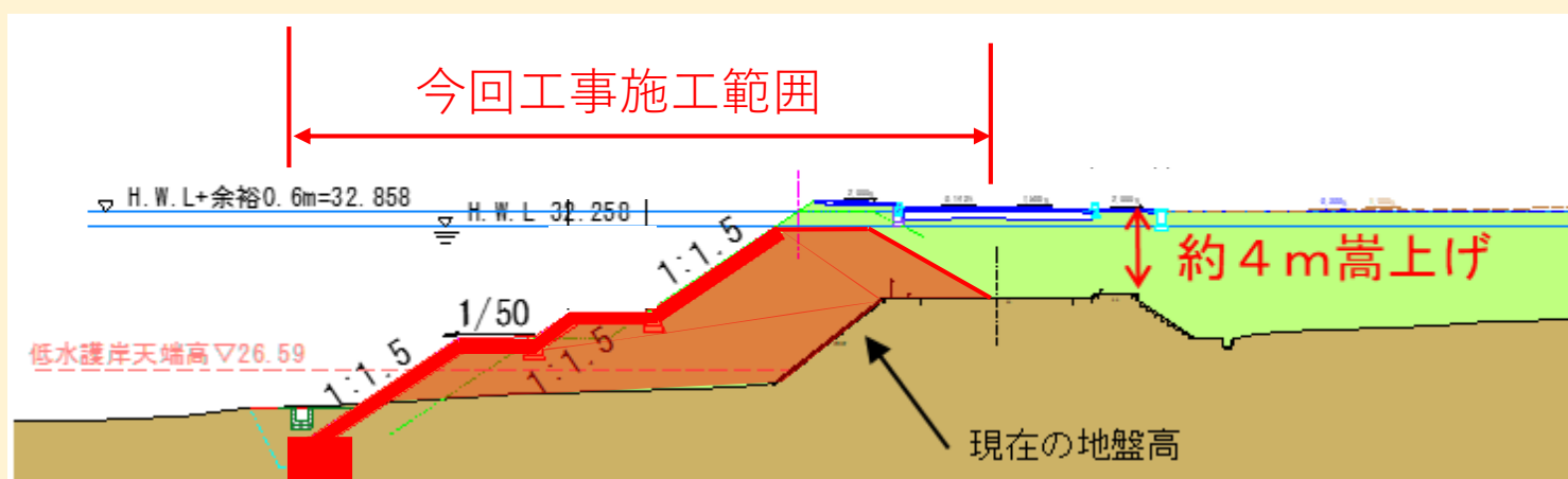
A-A 断面図
