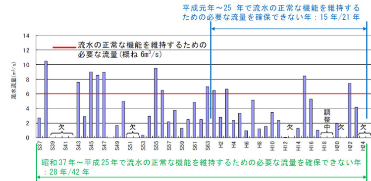
車尾地点における流況の経年変化
