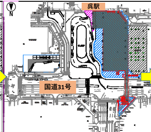
施工STEP④
