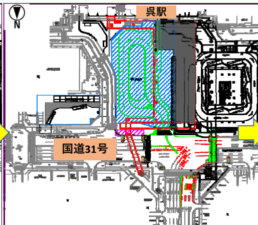
施工STEP⑦
