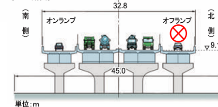
〔A-A'断面〕
