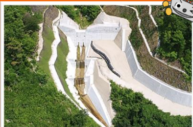
五月が丘4号砂防堰堤
