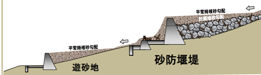
遊砂地イメージ
