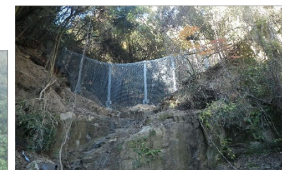
強靱ワイヤーネット設置状況
