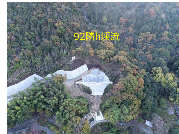
92隣h溪流 施工状況
