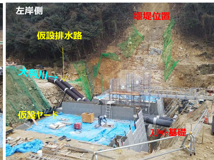
大判川打設状況（左岸側）
