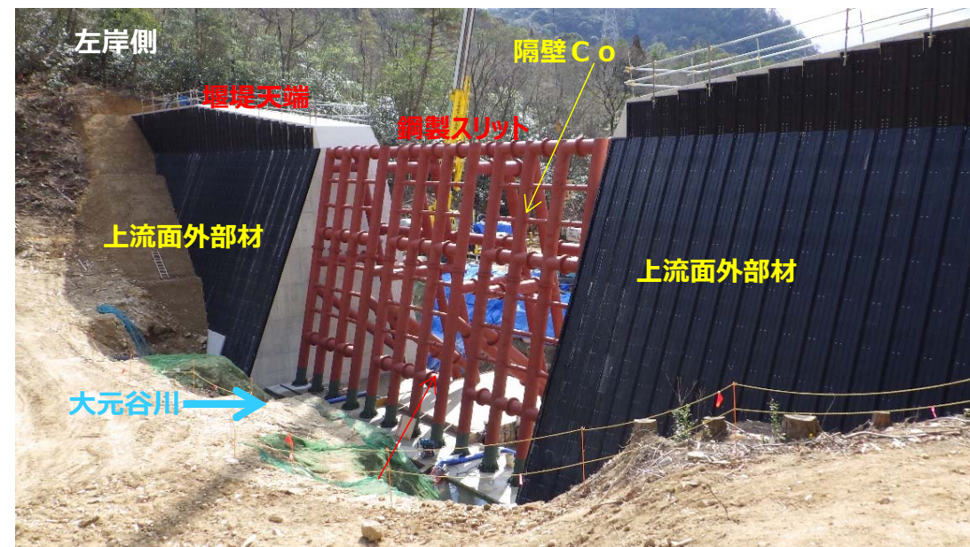
堰堤施工状況(上流側より)
