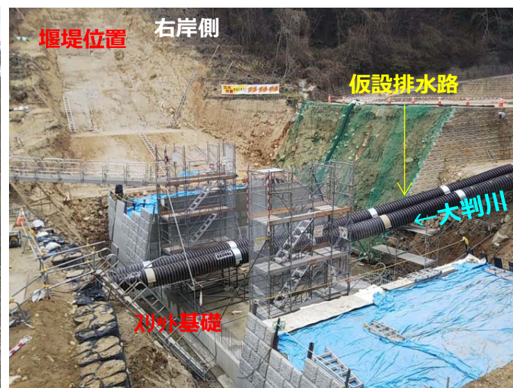
大判川打設状況（右岸側）
