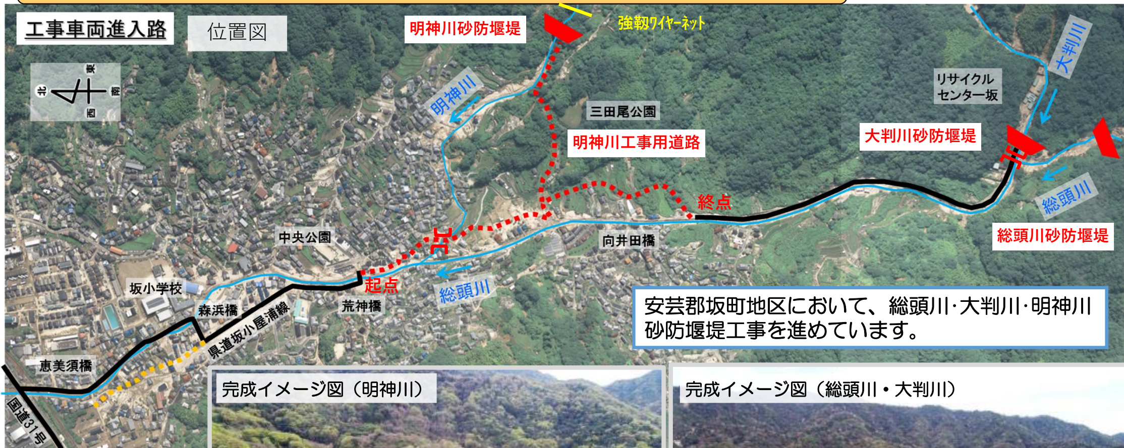
明神川砂防堰堤
