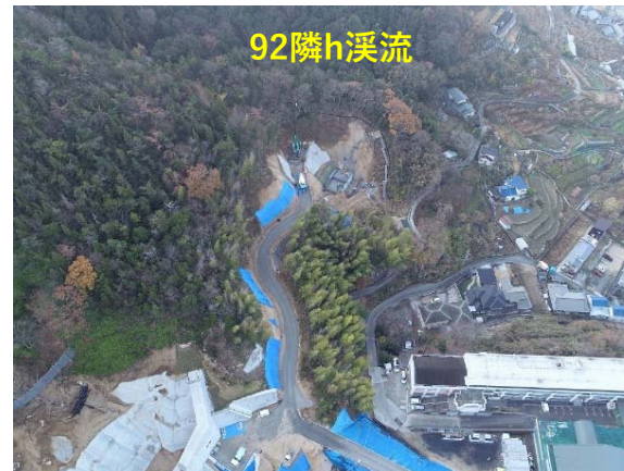
92隣h溪流 施工状況
