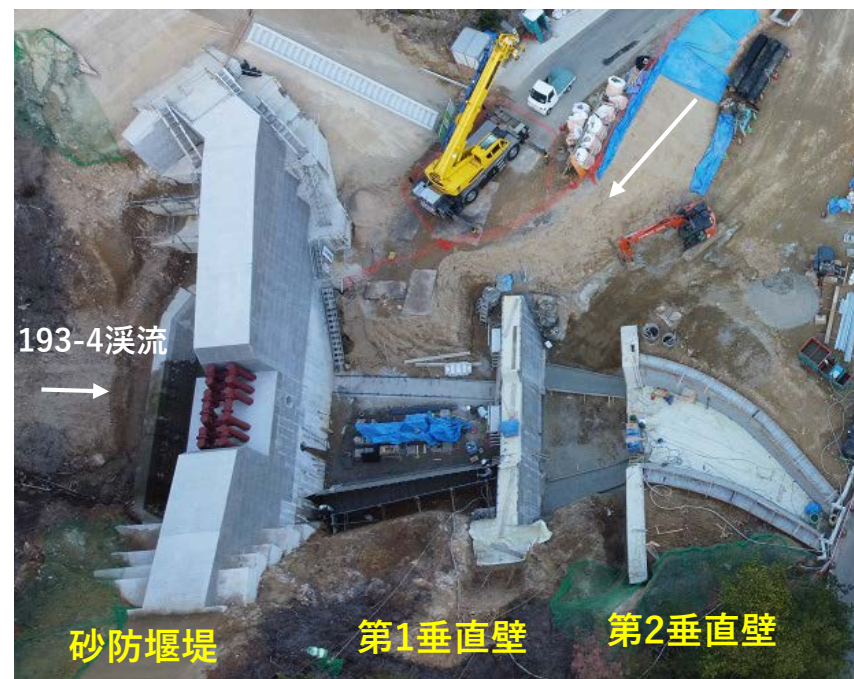
【施工状況（砂防堰堤、第1、2垂直壁）】
