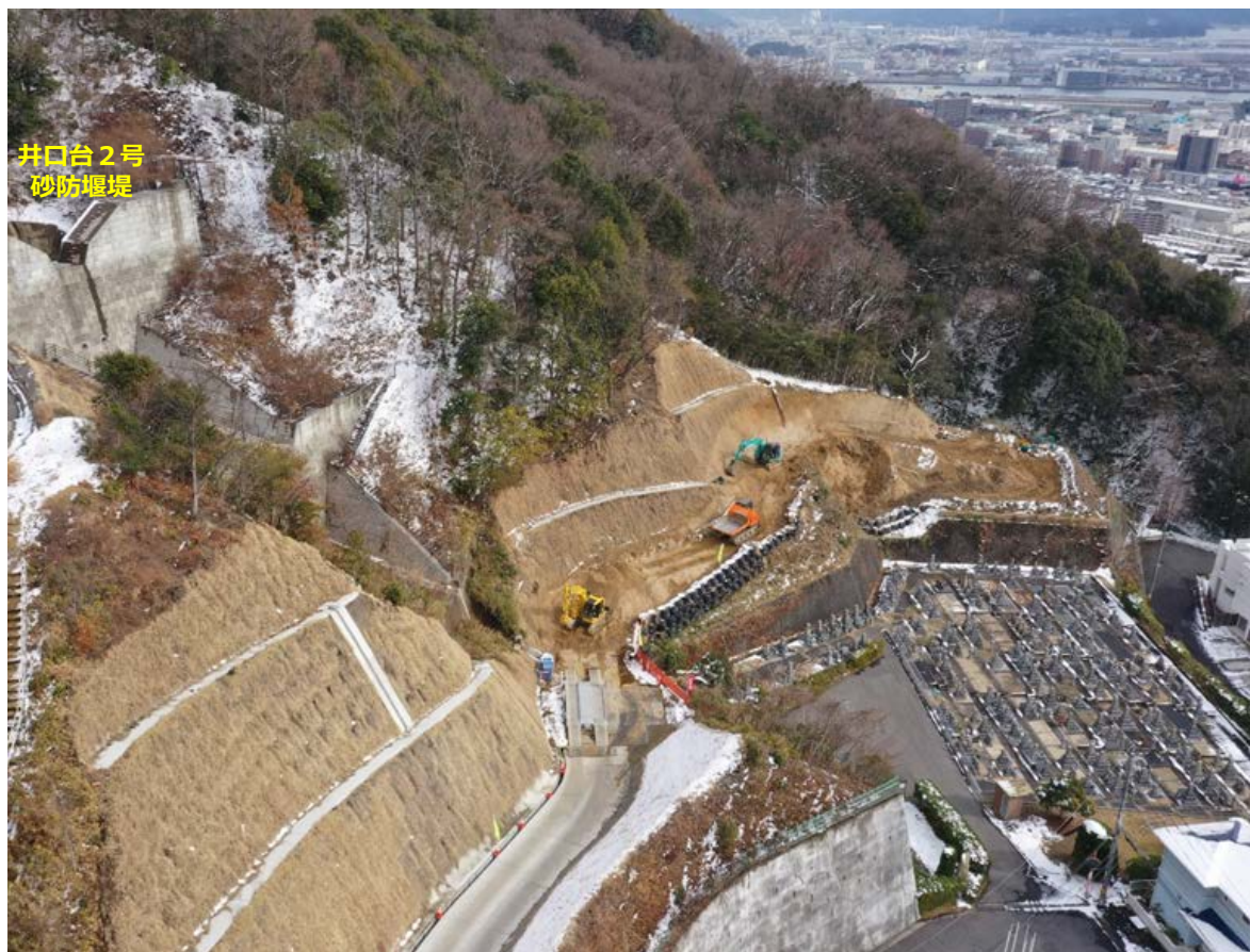
【全 景 (起点側より)】
