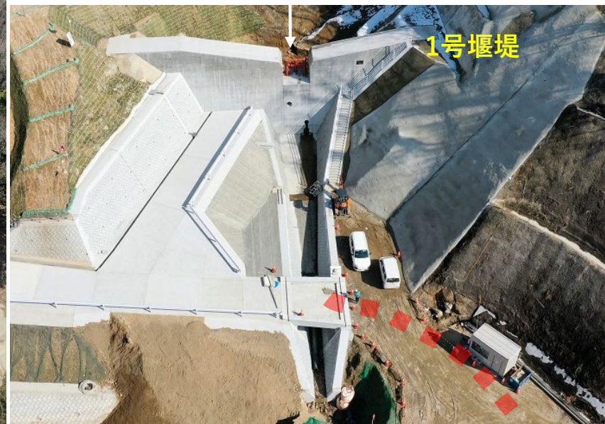
【1号堰堤 施工状況 (管理用道路)】
