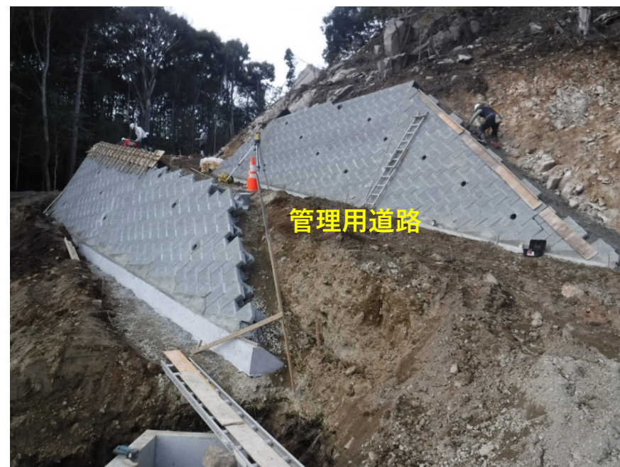
【施工状況 (管理用道路)】
