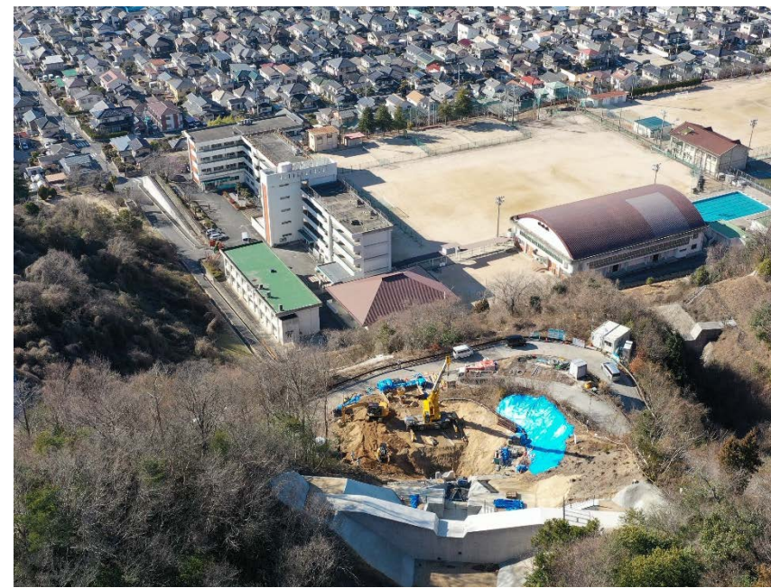
【砂防堰堤 施工箇所(上流側より)】
