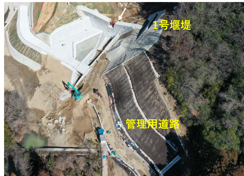
【1号堰堤 施工状況 (管理用道路)】
