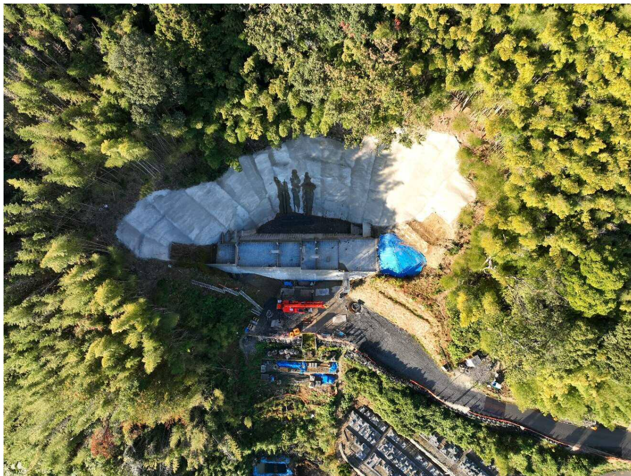
【施工状況】
