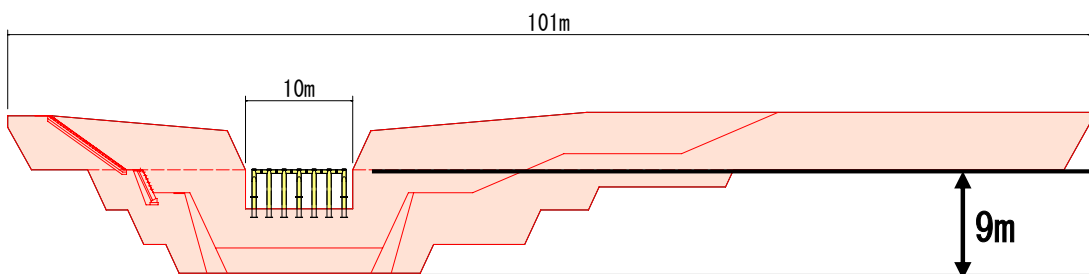
【砂防堰堤（本堤）正面図】
