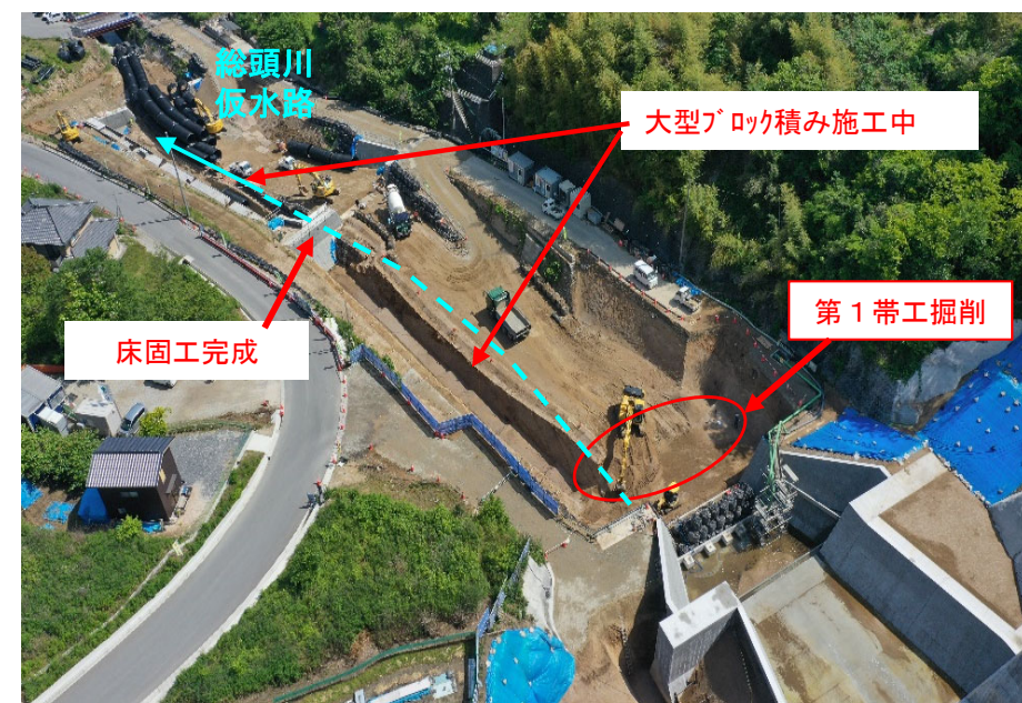
【大型ブロック積施工状況(上流から下流を望む)】
